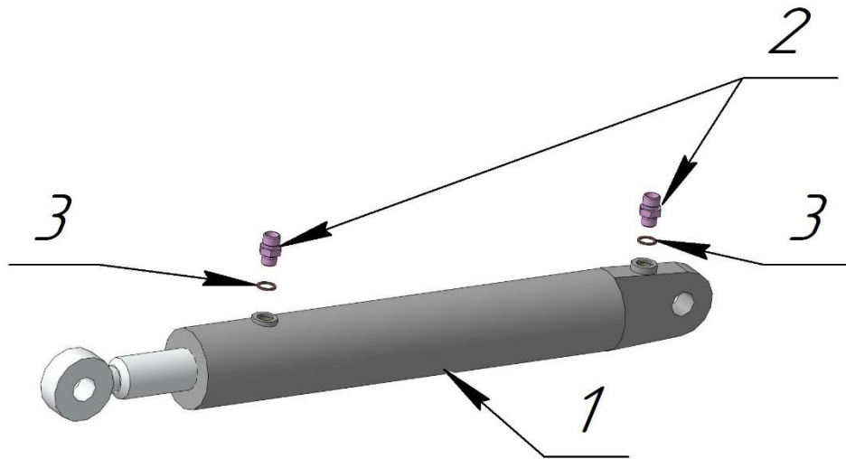
ГИДРОЦИЛИНДР (Рис. 11)
